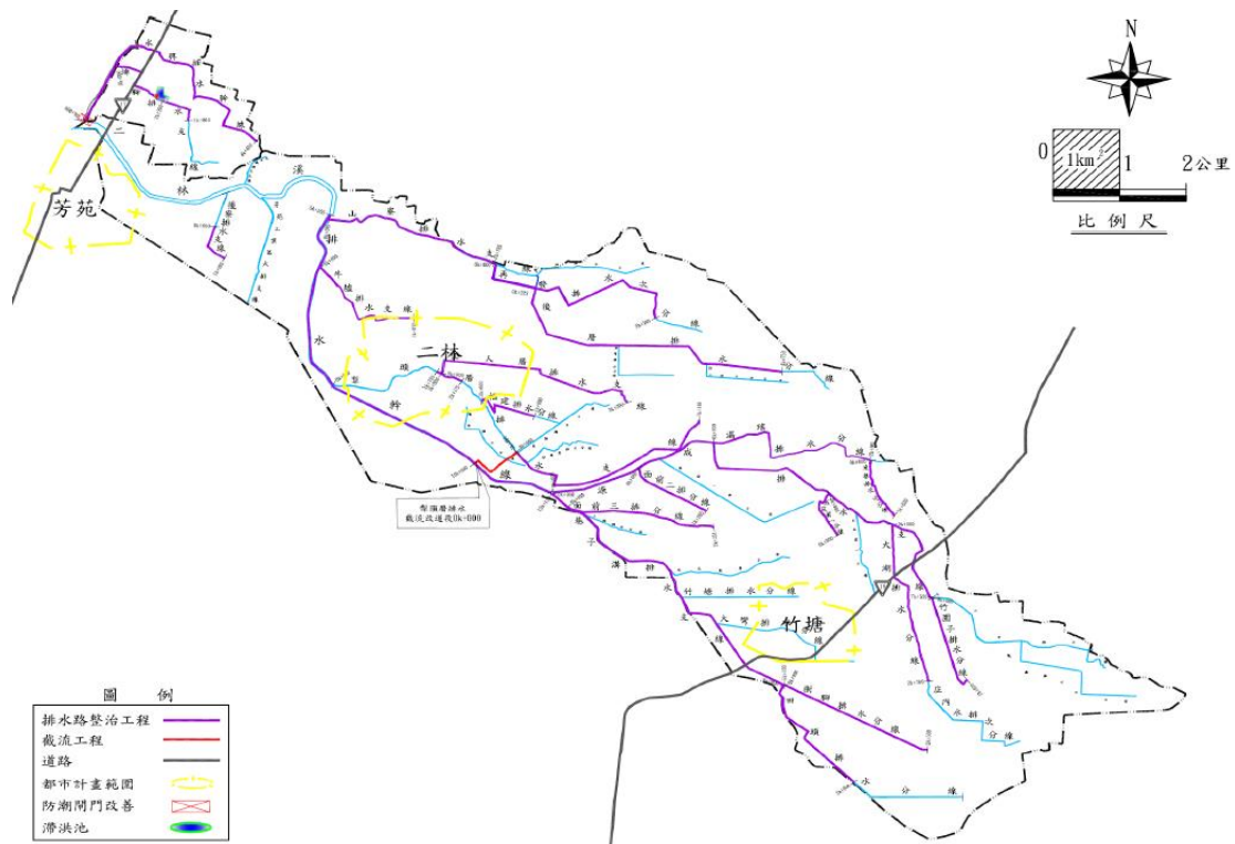
圖 2 埤腳排水改善工程佈置圖
