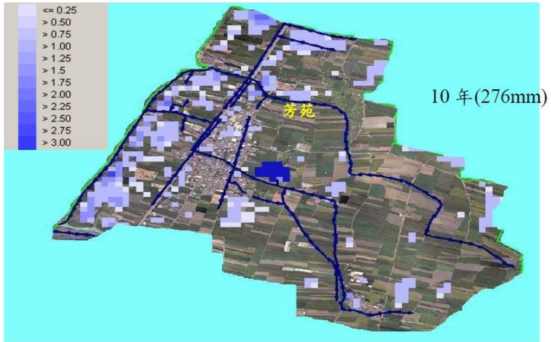
圖 3 埤腳排水改善重現期距 10 年淹水範圍
