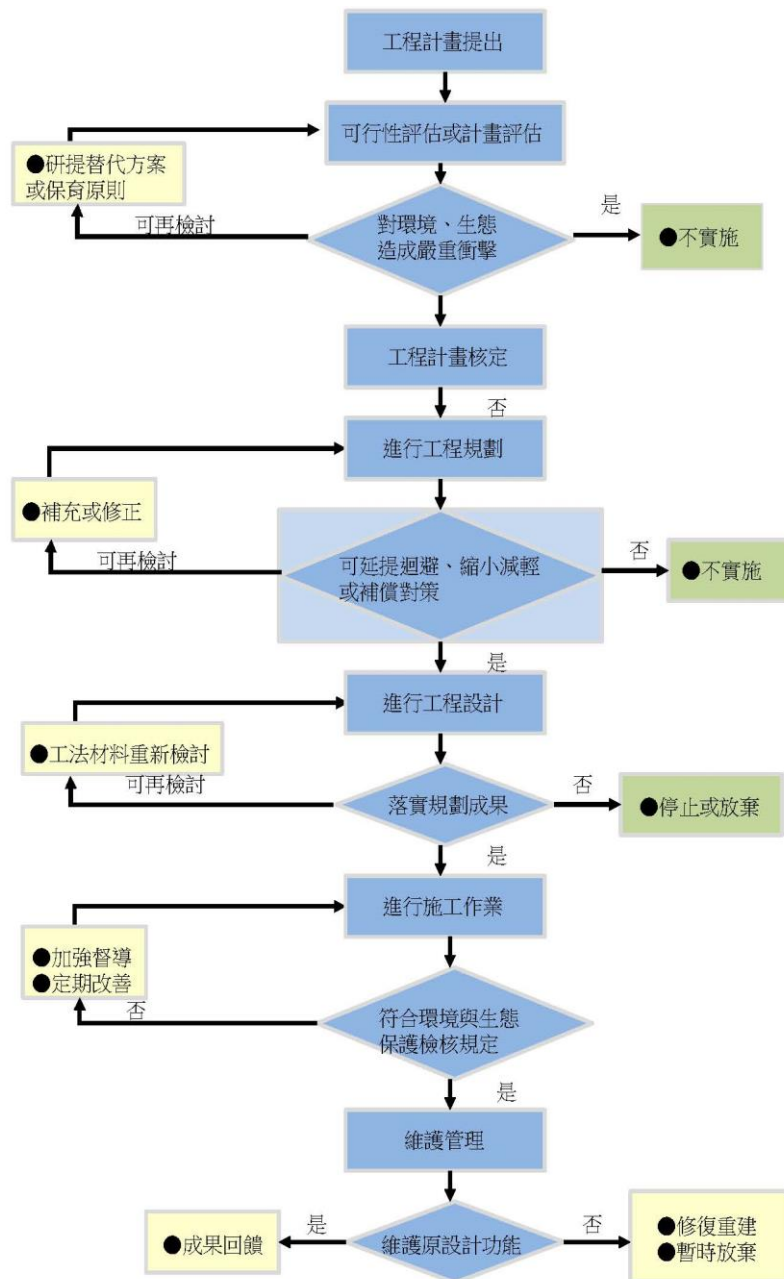
圖 3.1 公共工程生態檢核作業流程
