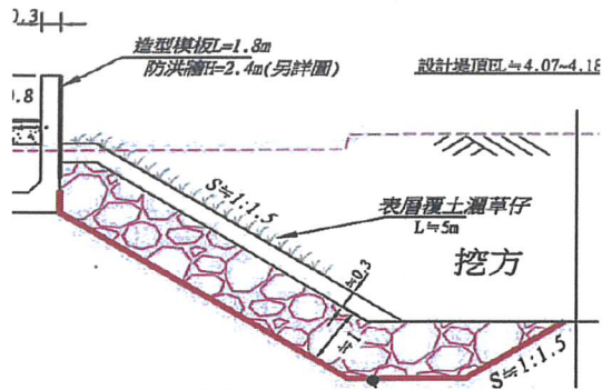
[設計圖]
