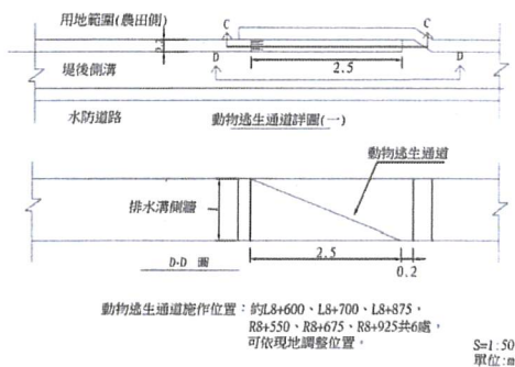
[設計圖]
