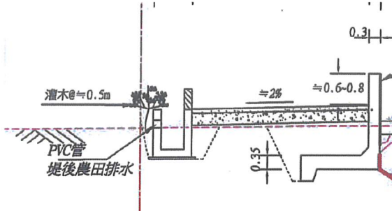
[設計圖]
