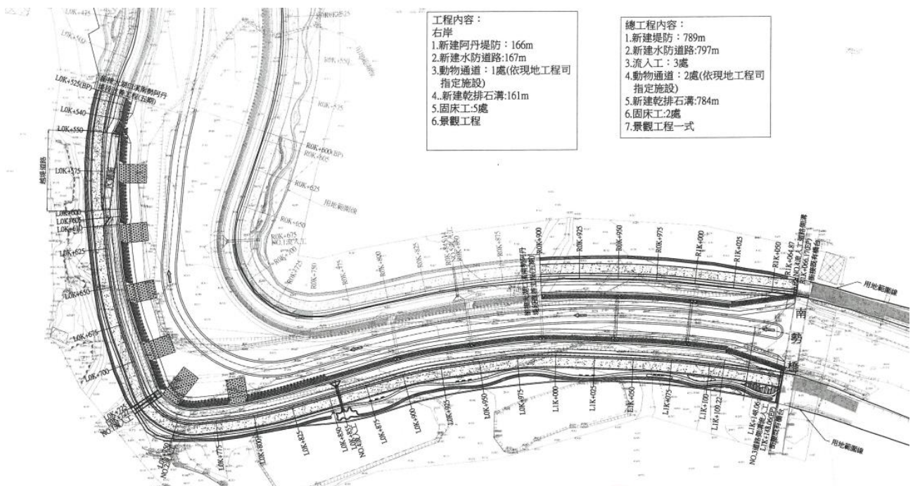
圖 3-1 工區設計圖
