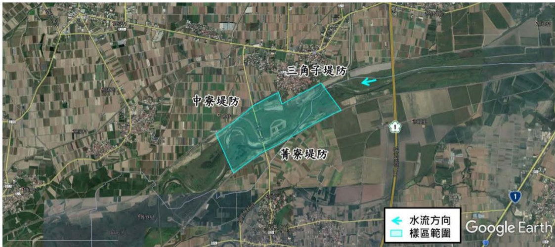
「八掌溪斷面 52~斷面 56」地理位置及堤防
