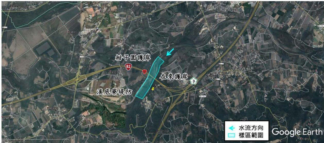
「赤蘭溪斷面 22~斷面 26」地理位置及堤防
