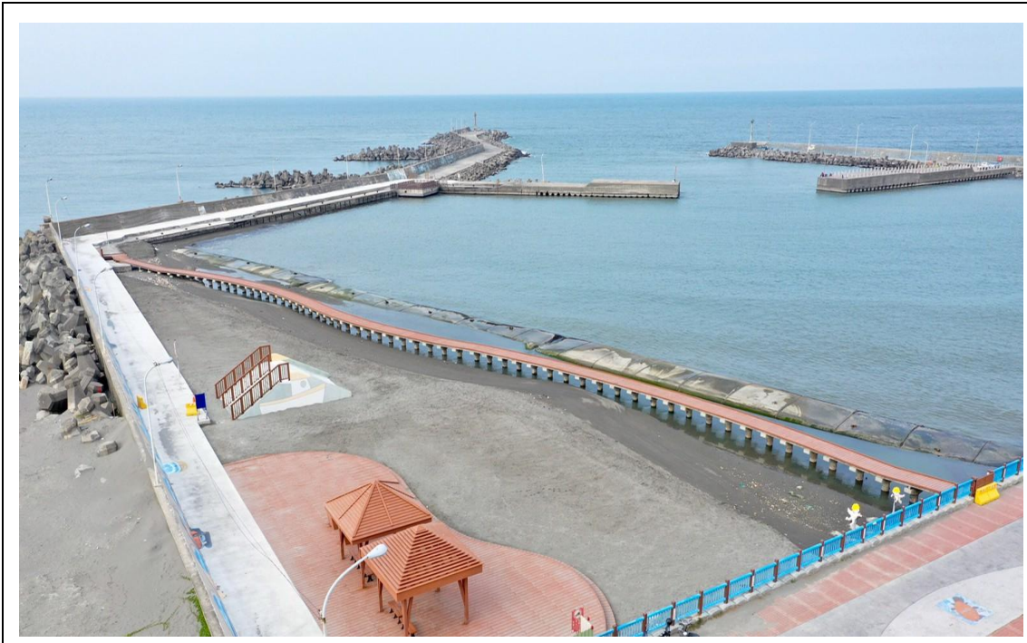
圖 2 堤防鋪面改善、人造灘地及水中廊道
