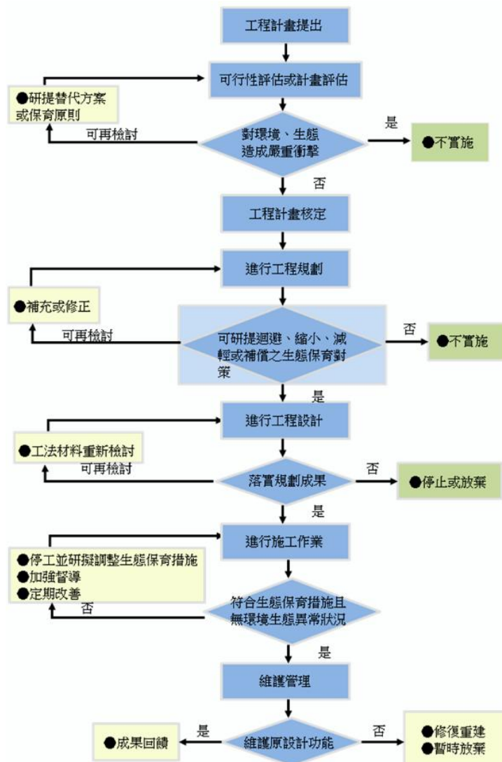
圖 8 公共工程生態檢核作業流程圖
