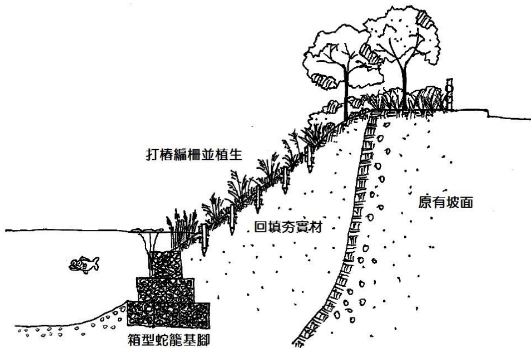
圖 4-1 崩塌地整治示意圖
