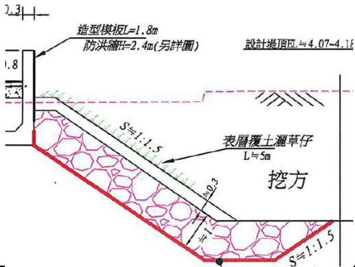
[設計圖]
