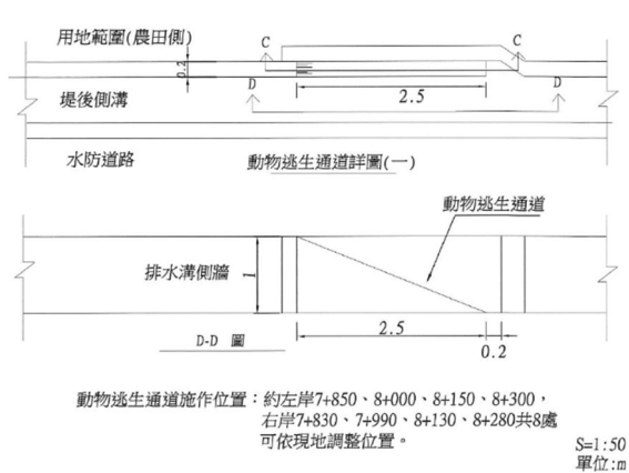
[設計圖]
