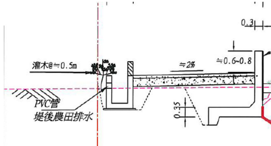
[設計圖]
